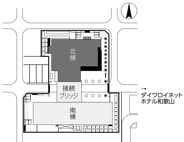
伏虎キャンパス平面図
